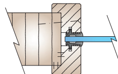
Glasausschnitt überfälzt
