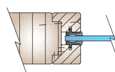
Glasausschnitt flächenbündig
